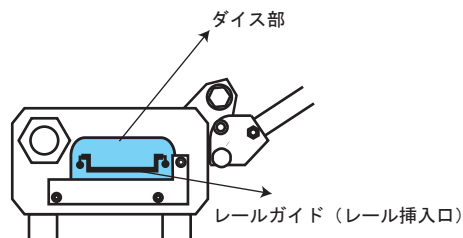
側面図
